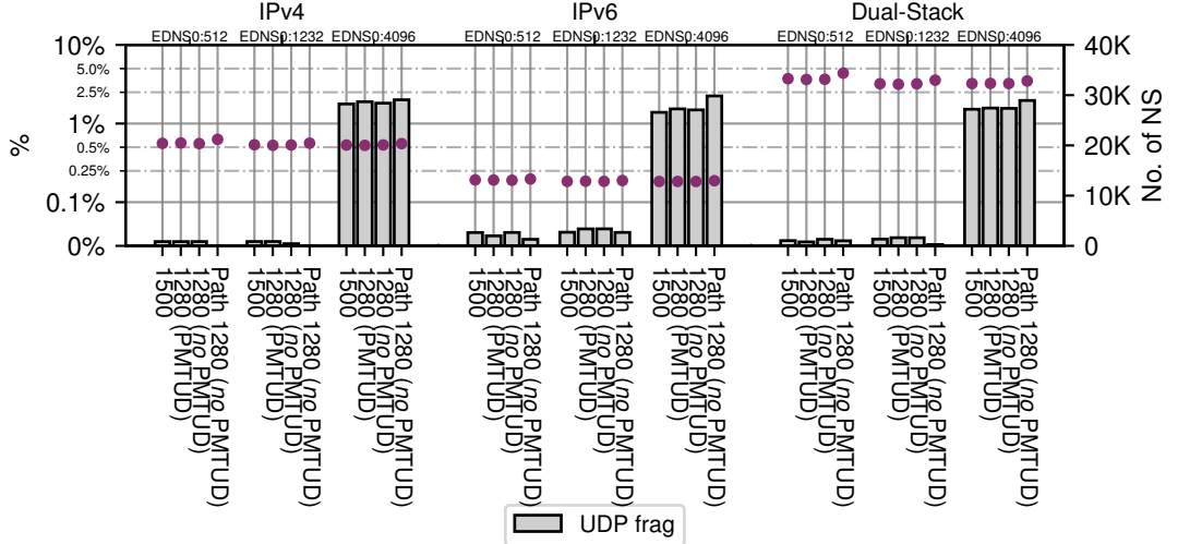
IPv4
