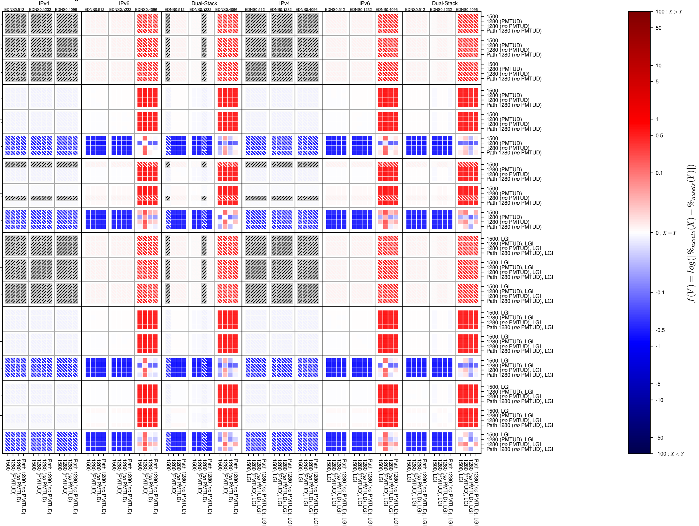
no_dnssec-v6-UDP_frag
