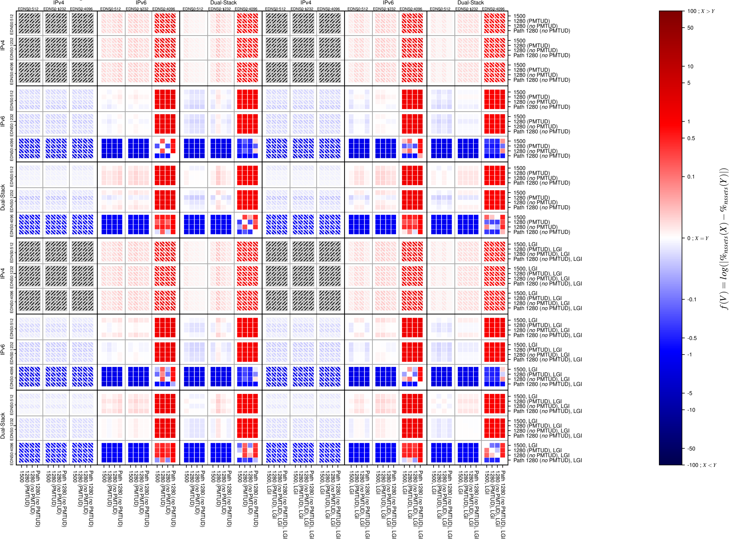
dnssec-v6-UDP_frag
