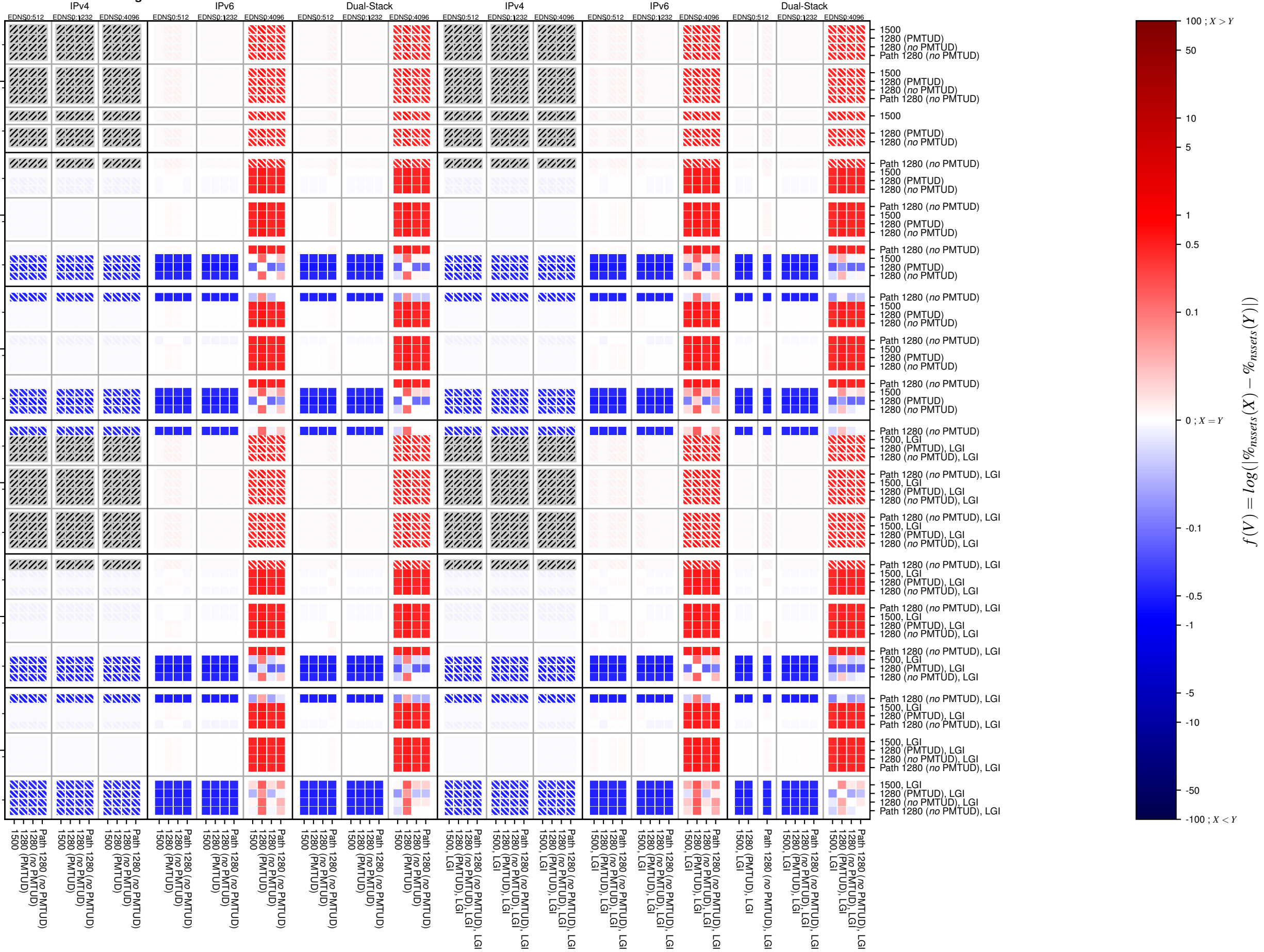
no_dnssec-v6-UDP_frag
